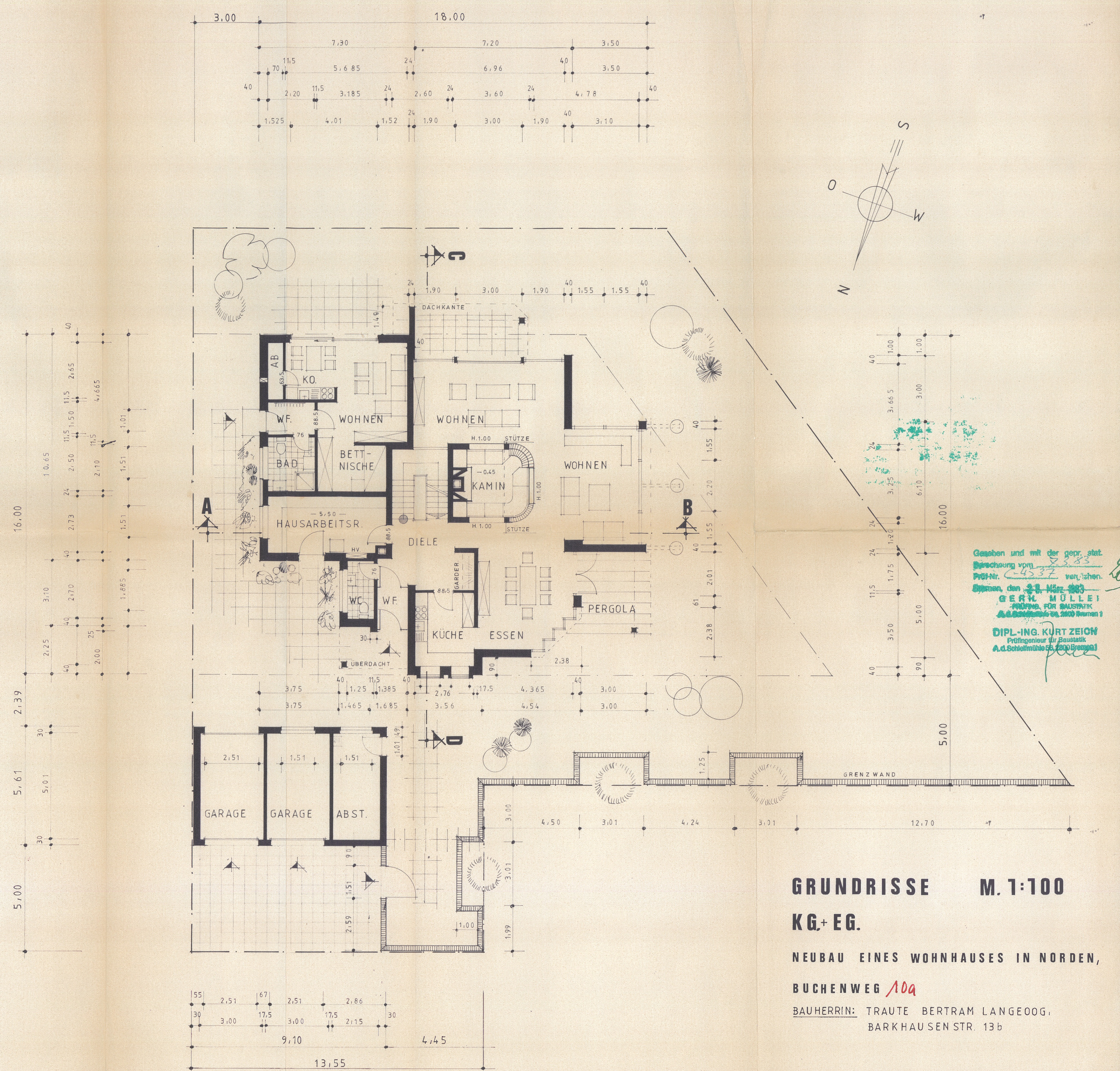
ERDGESCHOSS
