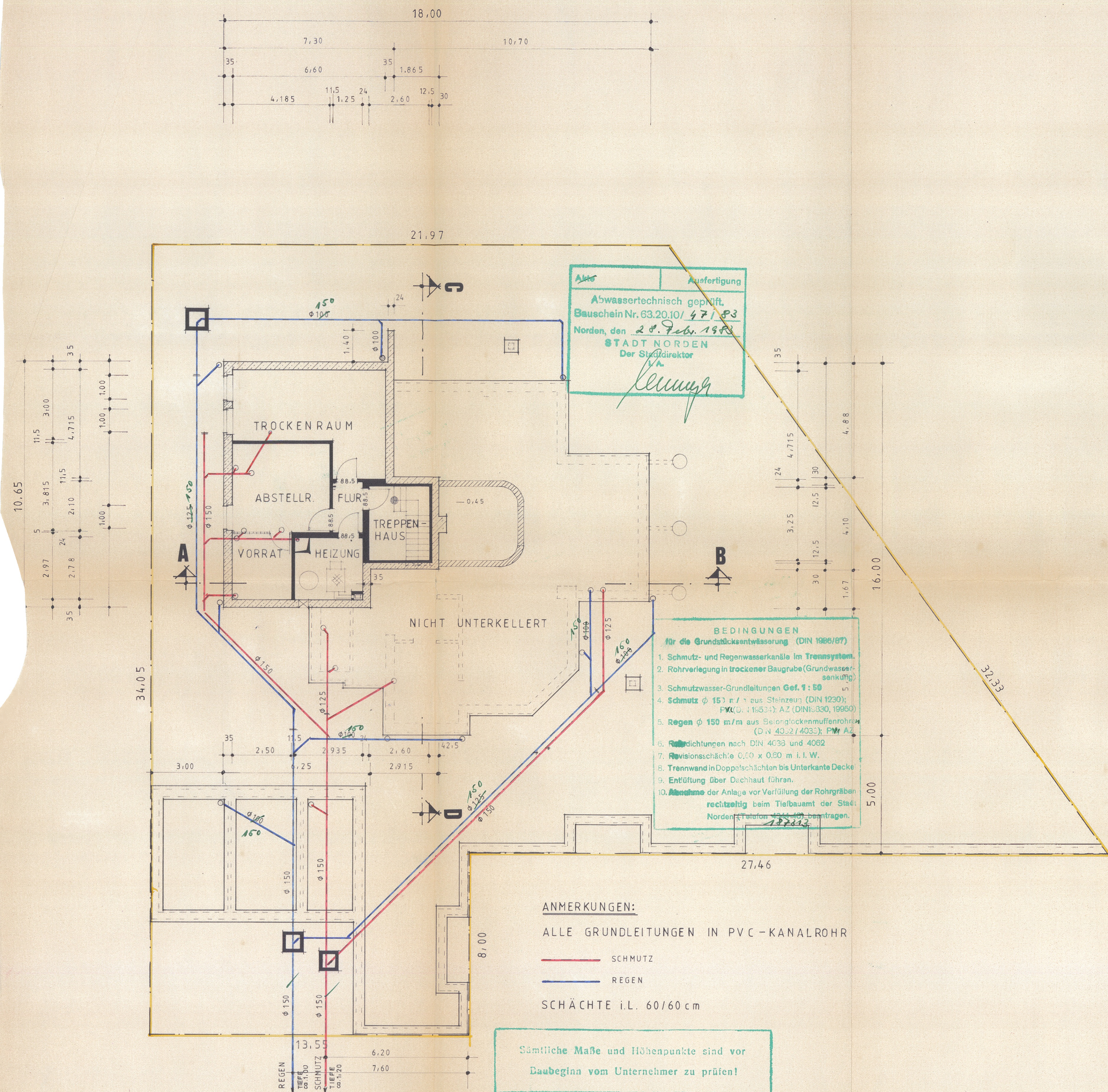
KELLERGESCH. + ENTWÄSSERUNG
